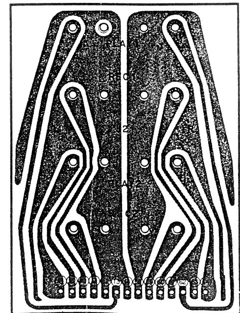
Tonbandgerät-Leiterplatte
